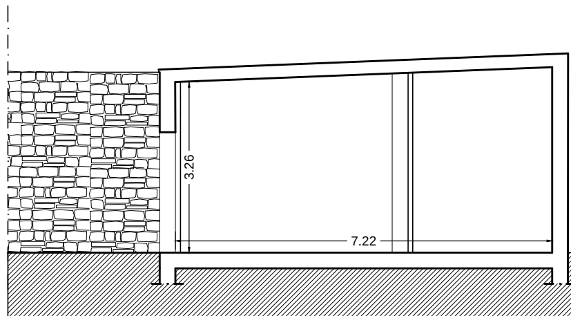
Sezione A-A
